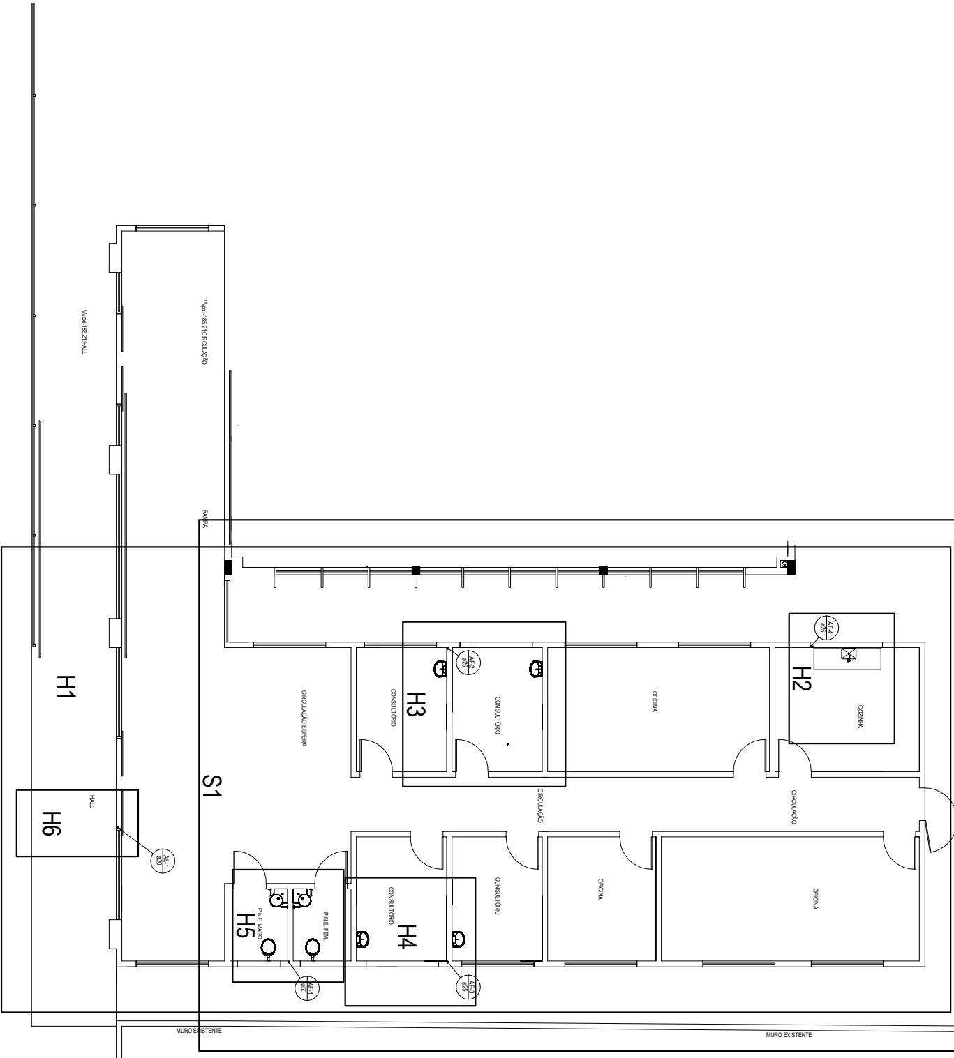
Croqui com Detalhes escala 1:25
